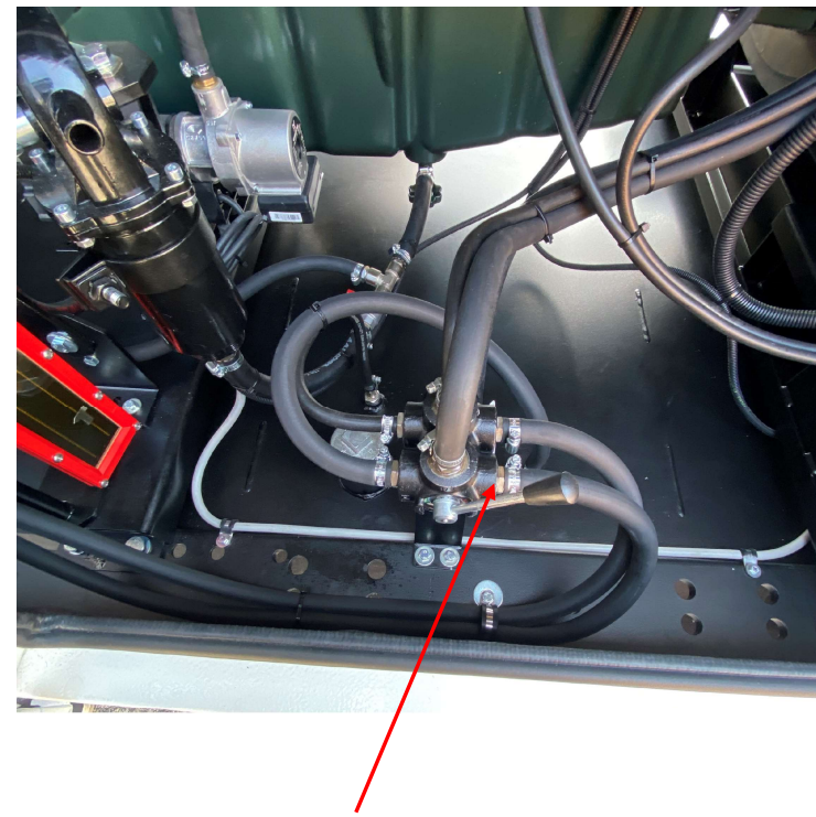
Valvula 3 vias para seleccionar el tanque interno o externo (Opcional)
